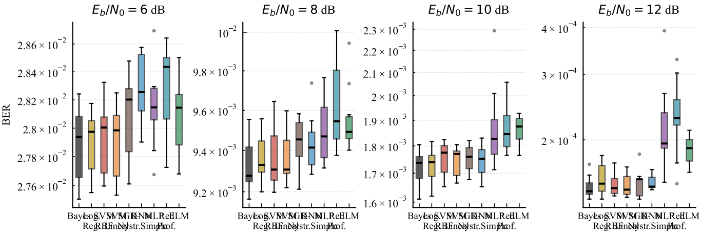
Distribución de BER por clasificador — E_b/N_0 clave
